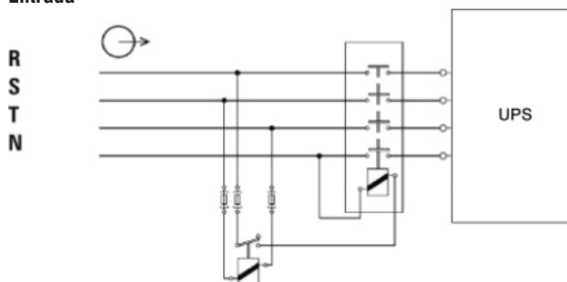
Figura 2-1: Conexiones de Protección contra Retroalimentación
