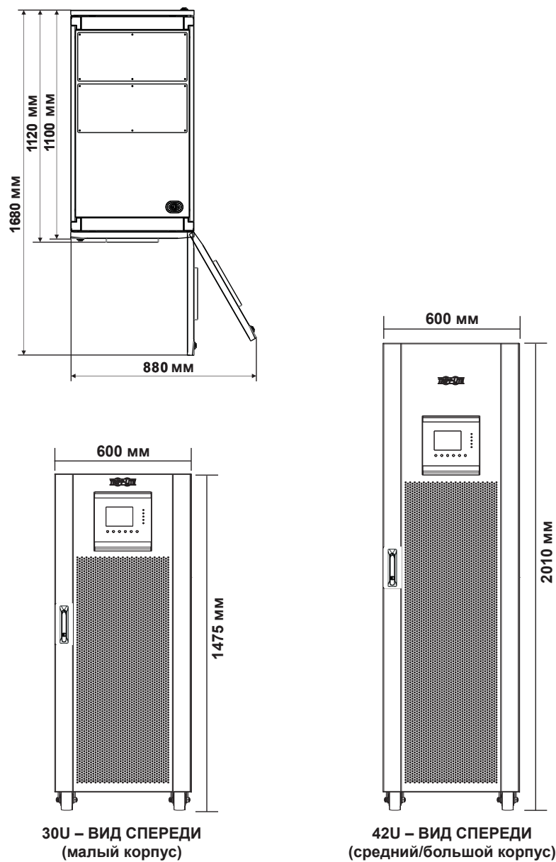
Рис. 3-1. Габаритные размеры
