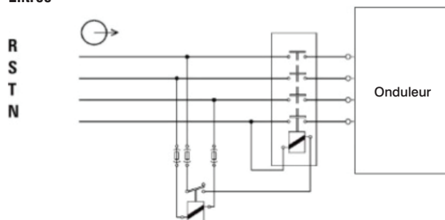
Figure 2-1 : Connexions de la protection de retour
