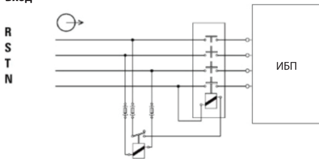
Рис. 2-1. Подключение устройства защиты от обратных токов
