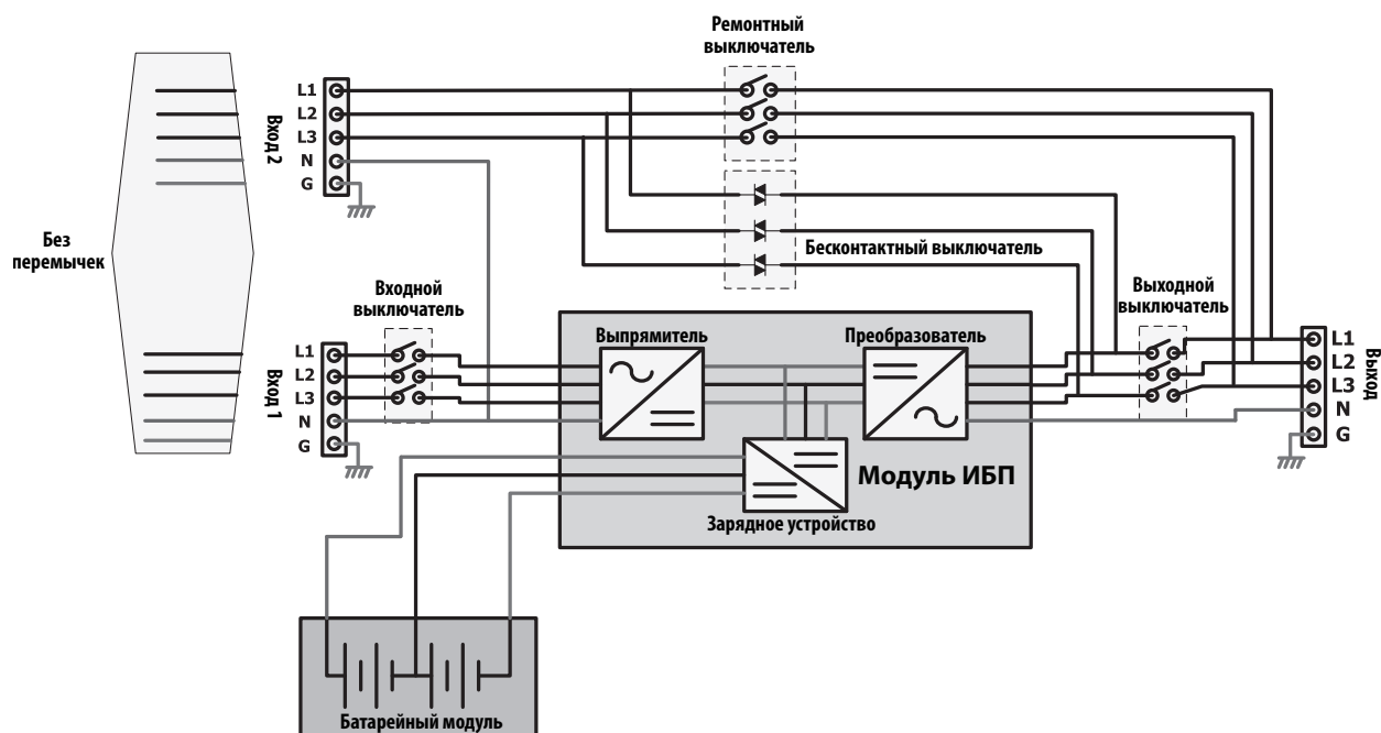
Рис. 5.1. Электрическая схема для двояного входа
