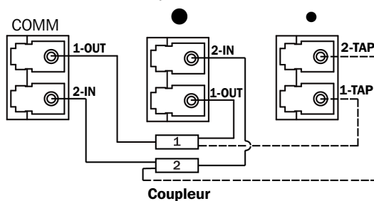
Schéma du port TAP de LC à LC
