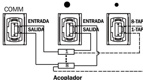
Mapeo de puerto TAP MPO a MPO
