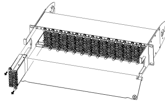
Étape 2. Insérer/retirer les cassettes TAP dans le/du panneau.
