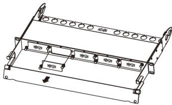
Schritt 1. Einlegen/Entfernen einer leeren Platte.
