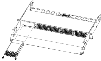
Schritt 2. Einlegen/Entfernen der TAP-Kassetten in das bzw. aus dem Panel.
