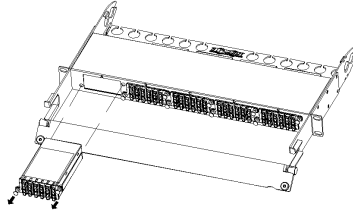
Étape 2. Insérer/retirer les cassettes TAP dans le/du panneau.
