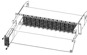
Шаг 2. Установка/извлечение TAP-кассет в панель/из панели.
