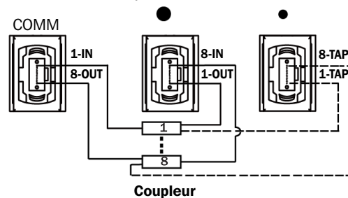
Schéma du port TAP de MPO à MPO
