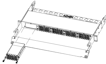
Paso 2. Inserción/extracción de casetes de TAP en el panel.
