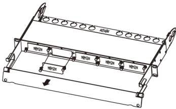
Étape 1. Insérer/retirer la plaque vide.
