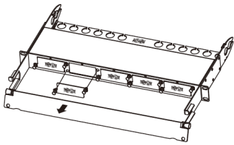
Шаг 1. Установка/извлечение заглушки.
