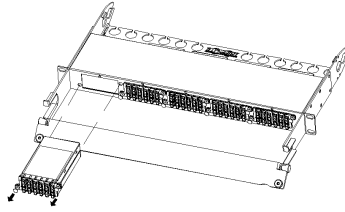
Шаг 2. Установка/извлечение TAP-кассет в панель/из панели.
