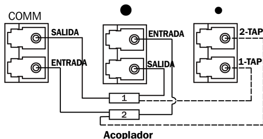
Mapeo de puerto TAP LC a LC
