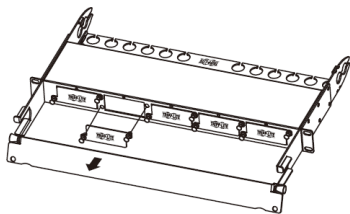
Paso 1. Inserción/extracción de la placa de obturación.
