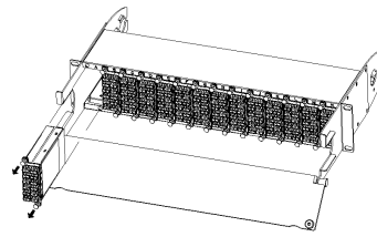
Paso 2. Inserción/extracción de casetes de TAP en el panel.
