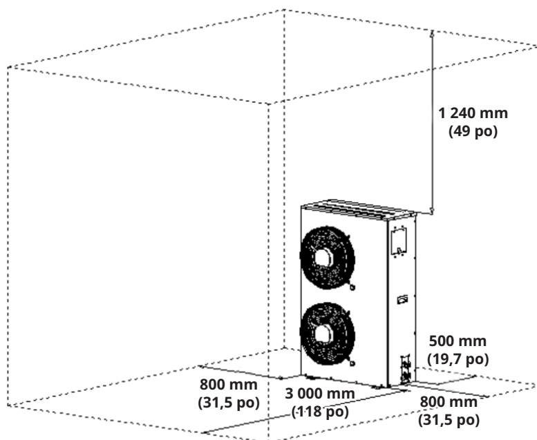
Figure 3-4A : Exigences pour le dégagement de l'installation - Condensateur (SRCOOLDXRW12)
