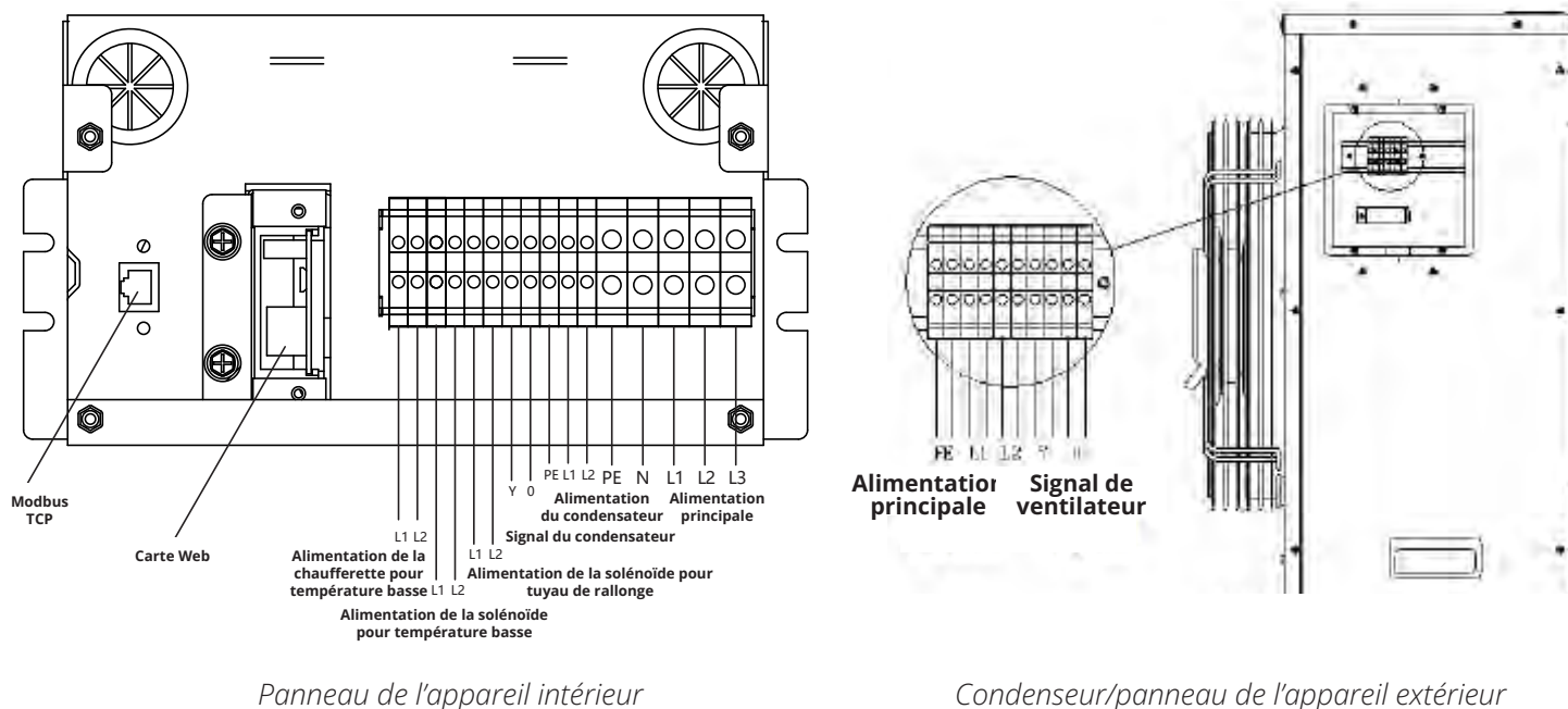
Figure 5-1a : Connexions électriques, SRCOOLDXRW12
