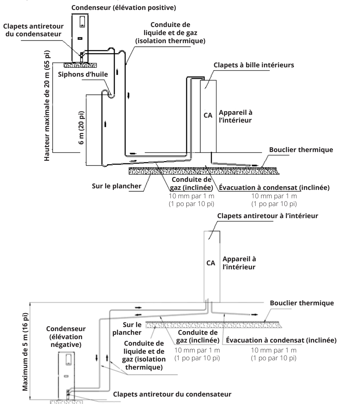
Figure 4-1 : Exemples de canalisations
