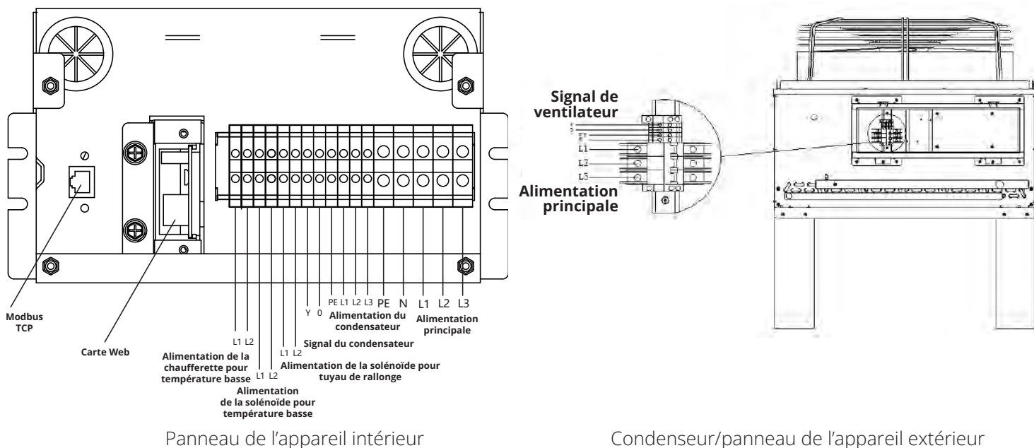
Figure 5-1b : Connexions électriques, SRCOOLDXRW25
