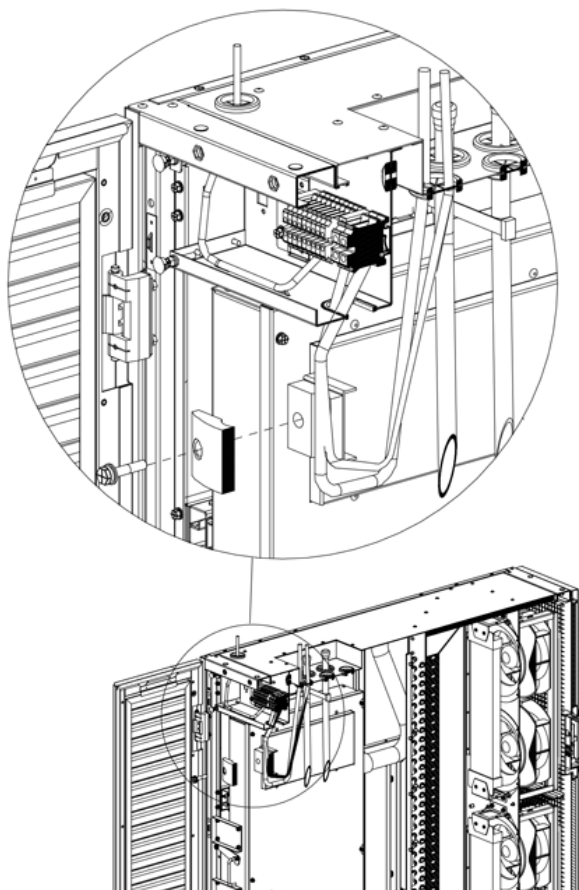
Figura 5-2A: Liberación de Tensión desde Arriba
