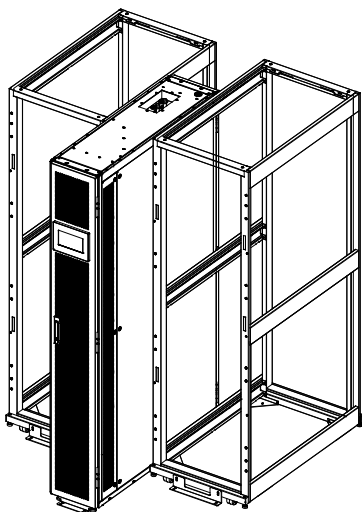
Figure 2-1 : Panneaux latéraux perforés installés, Airblock avant installé
