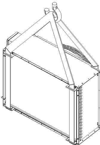
Figure 3-2 : Exemple de levage du condenseur
