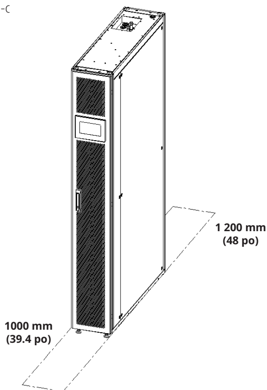
Figure 2-3 : Exigences pour le dégagement de l'installation
