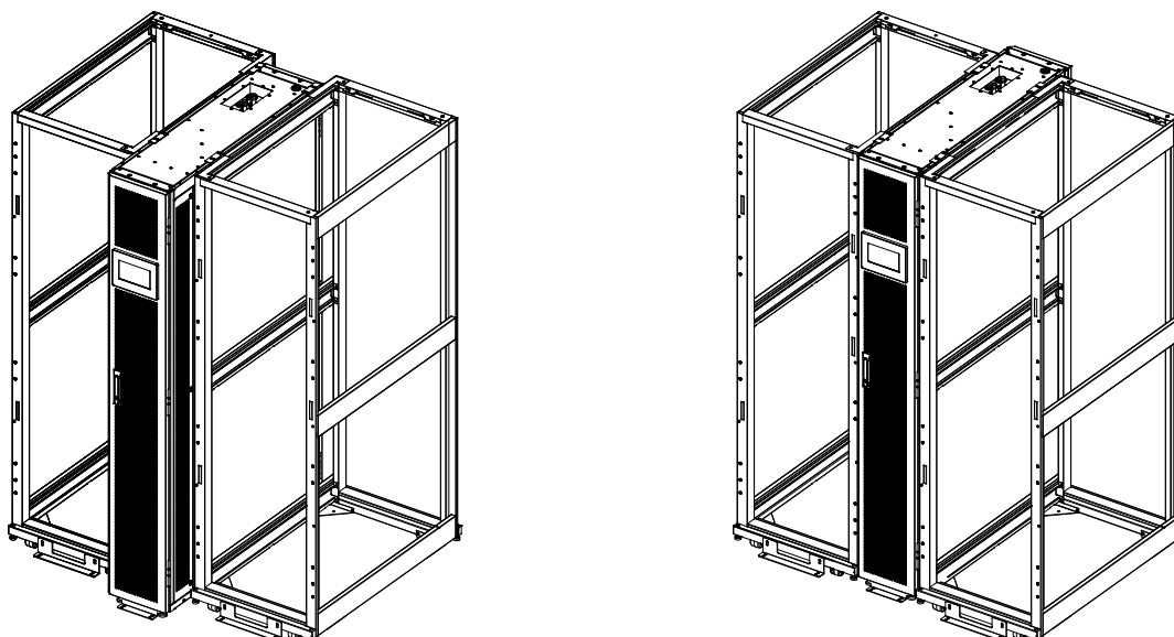
Figura 2-4: Instalación sobresaliente (izquierda) y a ras (derecha)
