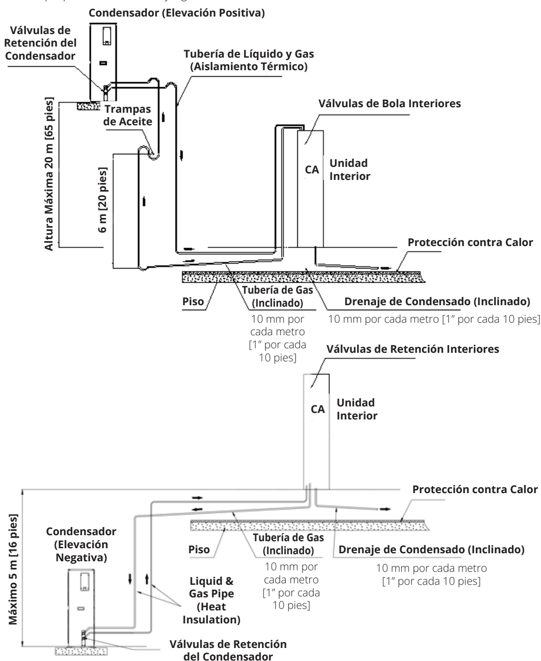
Figura 4-1: Ejemplos de Tubería
