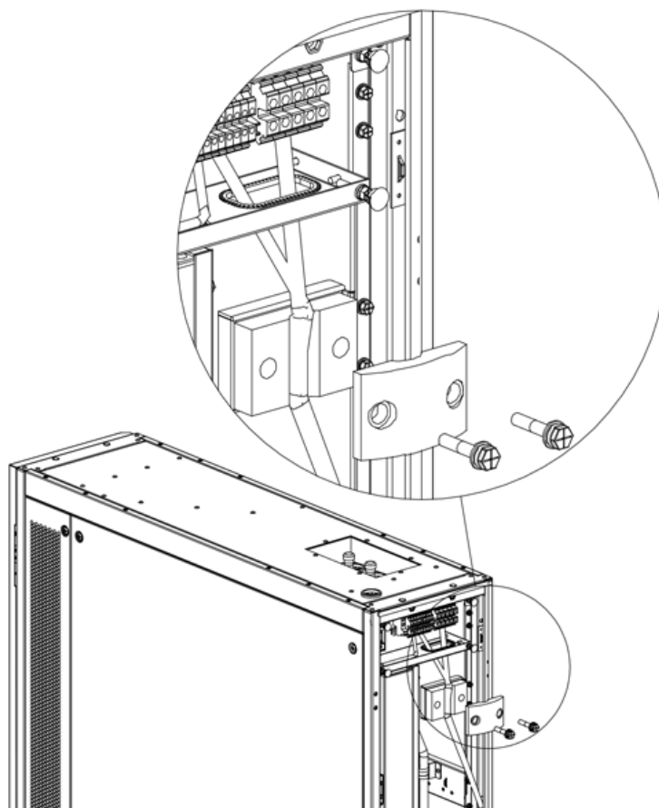
Figura 5-2B: Liberación de Tensión desde Abajo
