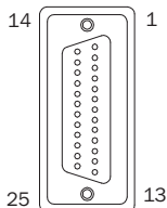
ANSCHLUSS.1 DB25-STECKER
