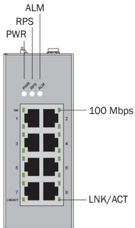
Frontansicht
