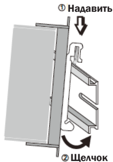
Крепление коммутатора
